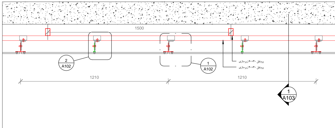
برش افقی ۱ ۱ : ۱۰ 0 10 20 40
