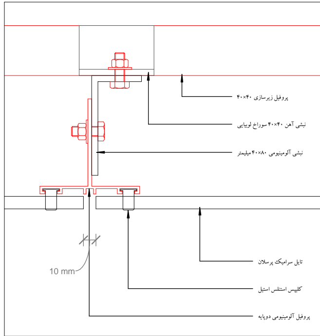
۱ جزئیات اتصال مولیون اصلی ۱ : ۲
