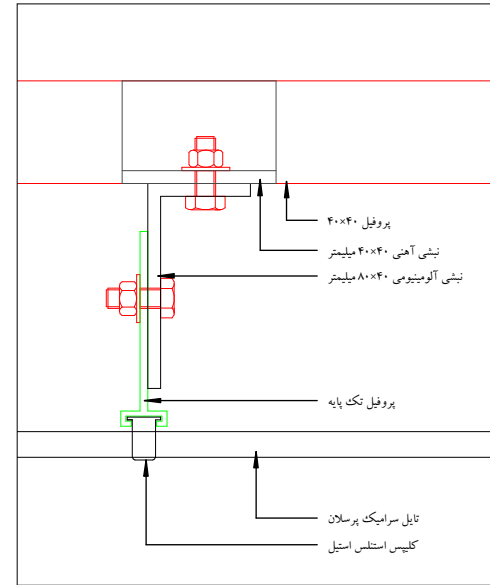
۲ جزئیات اتصال مولیون فرعی ۱ : ۲
