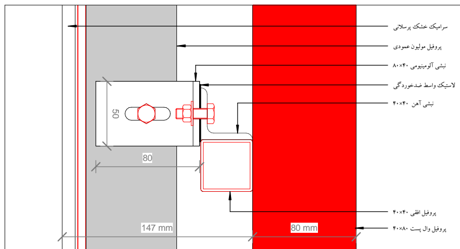
بزرگنمایی اتصال مولیون ها ۲ : ۱
